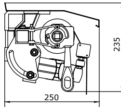
Homlokzati rögzítés védőtetővel
