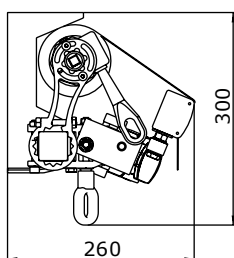
Mennyezeti rögzítés
