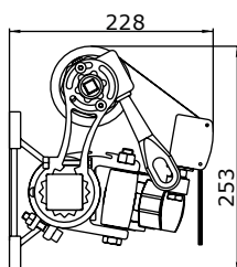
Homlokzati rögzítés
