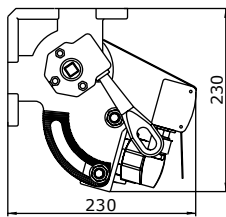
Univerzális rögzítés
