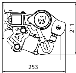
Homlokzati rögzítés
