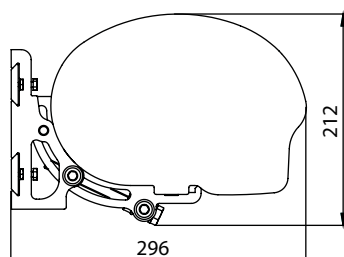
Homlokzati rögzítés
