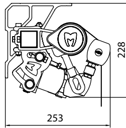
Univerzális rögzítés
