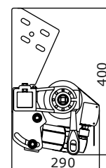
Szarufa rögzítés
