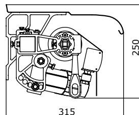
Homlokzati rögzítés védőtetővel
