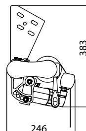
Szarufa rögzítés
