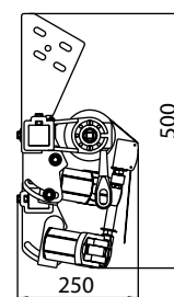
Szarufa rögzítés
