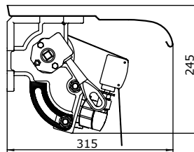
Homlokzati rögzítés védőtetővel
