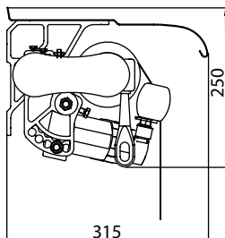
Homlokzati rögzítés védőtetővel
