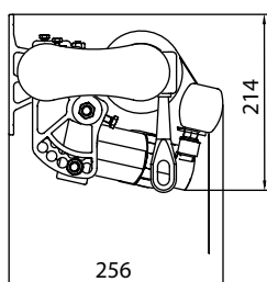
Homlokzati rögzítés
