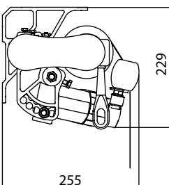
Univerzális rögzítés
