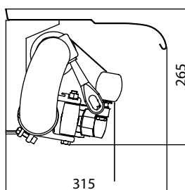
Homlokzati rögzítés védőtetővel
