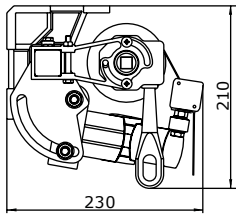
Univerzális rögzítés
